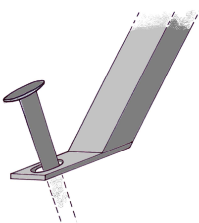
Patka panelu s ukotvením
